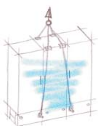
B. Schwerlastsocket mit Seilanschlagstangen (ca. 3 t)
