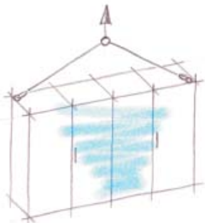
D. STARPOINT-Ringschrauben M16 (2 St. / 45° = 2,1 t)
