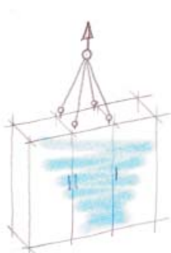
A. Ringschrauben M16 (4 St. / 60° = 1,3 t)
